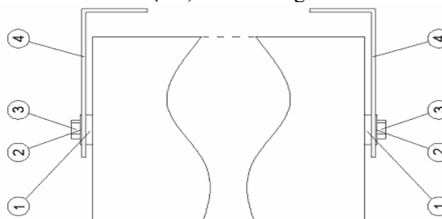
Fig. 1 – Prinderea colțarelor
