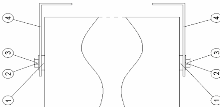
Fig. 4 – Prinderea colțarelor
